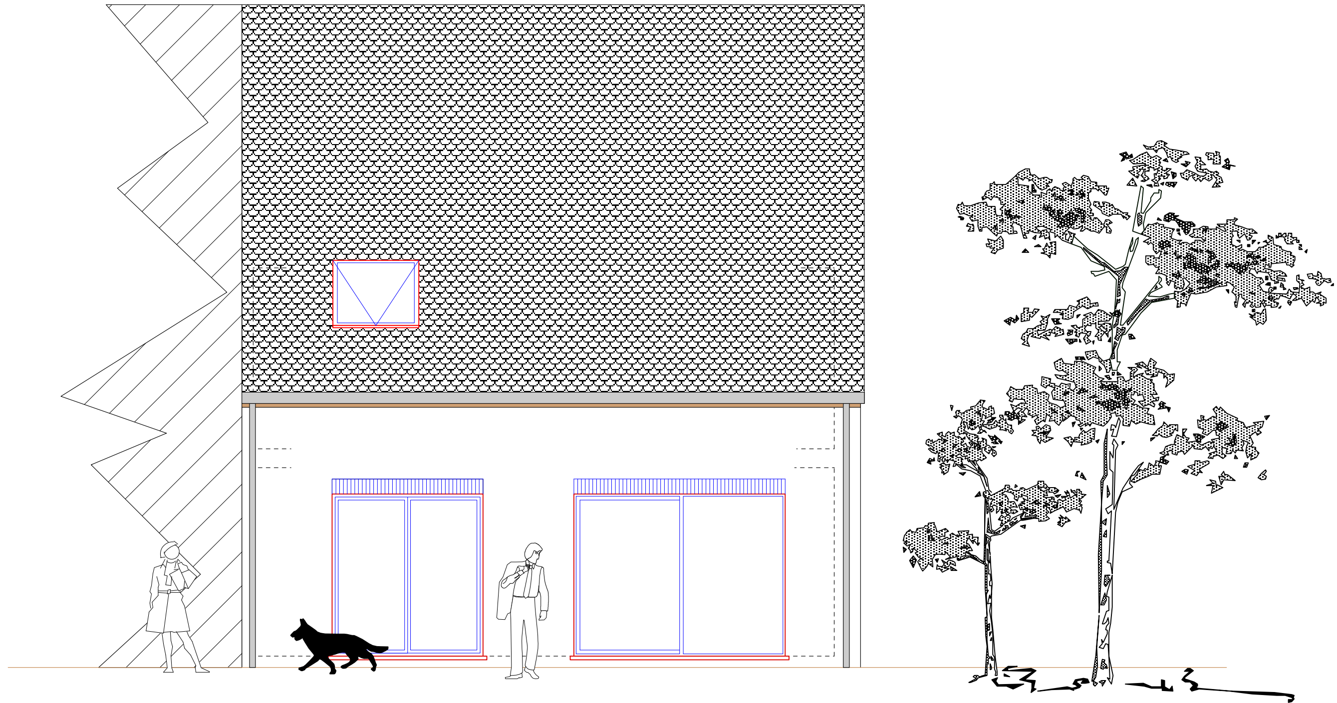
ACHTERGEVEL
